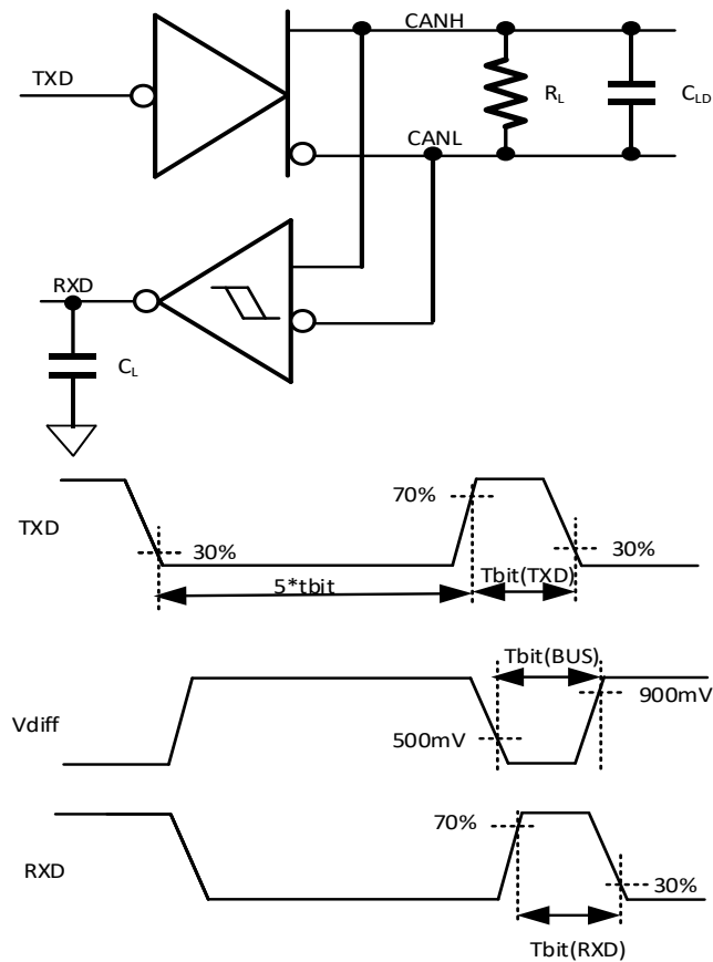
图 10-4 CAN FD 时序示意图
