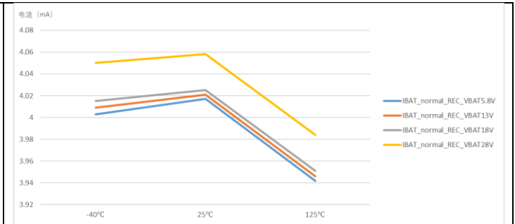
图 9-2 隐性状态电流
