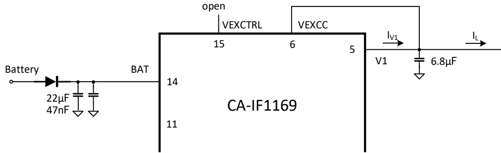
图 11-3 V1 在内部供电
