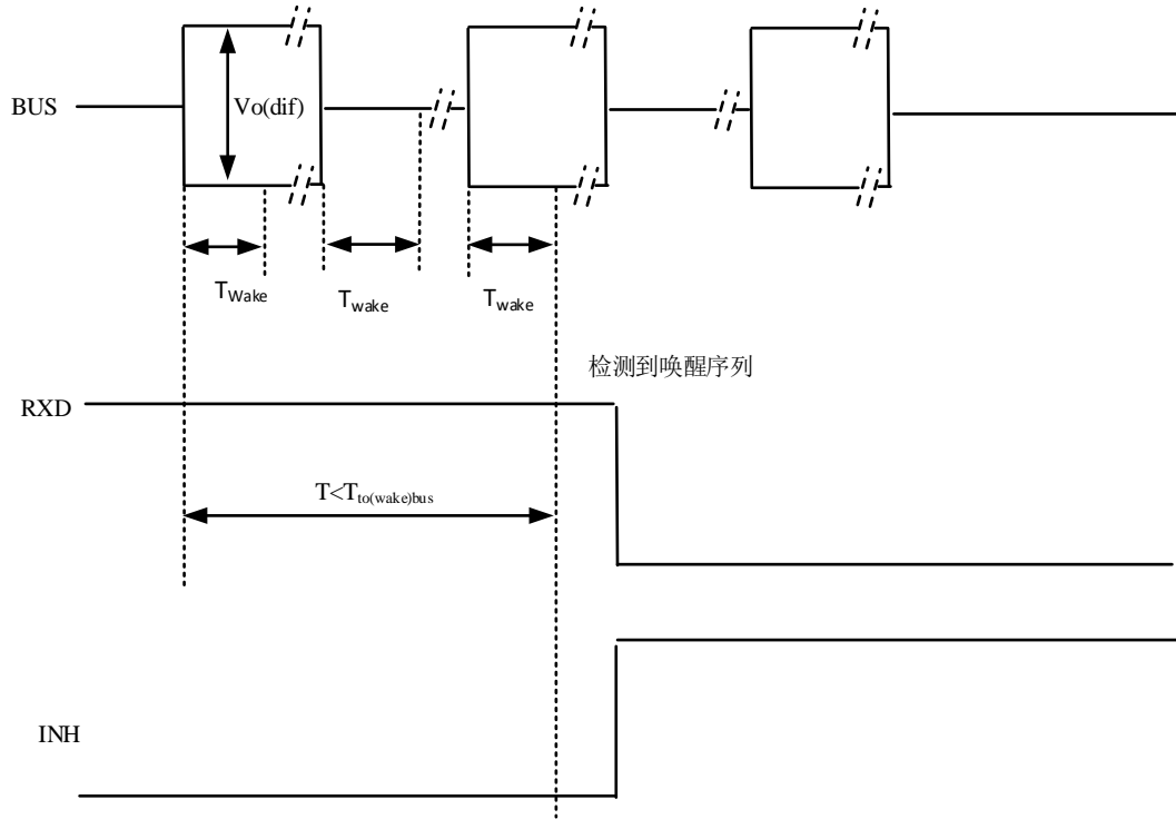
图 11-8 总线唤醒序列示例图
