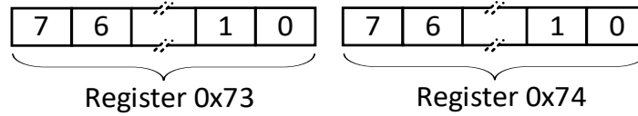
图 11-13 CRC 计算的数据表示
