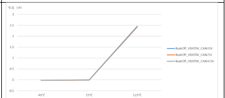
图 9-4 BusFault 电流
