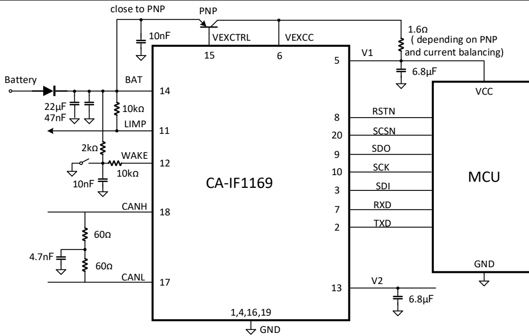
图 12-1 CA-IF1169 的典型应用图
