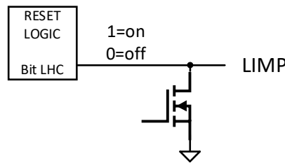
图 11-6 LIMP 管脚电路图
