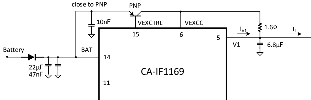
图 11-4 V1 在内部与外部 PNP 共同供电
