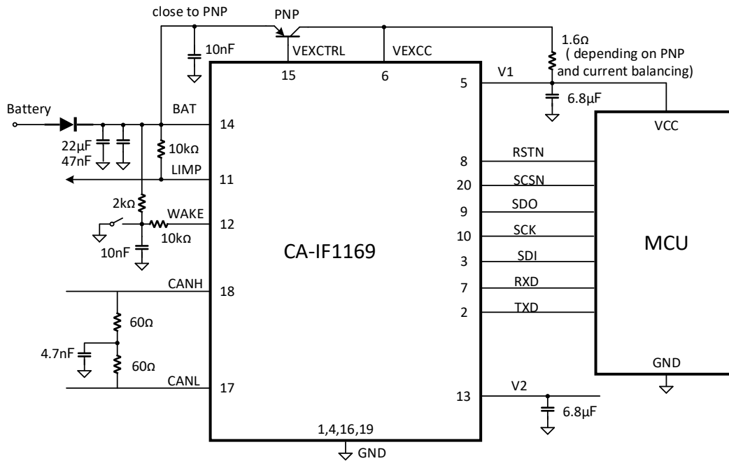
典型应用框图
