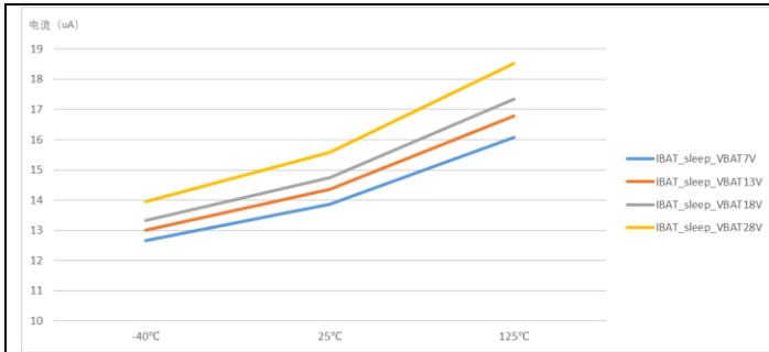
图 9-1 静默态电流
