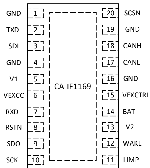
图 8-1 CA-IF1169 引脚图
