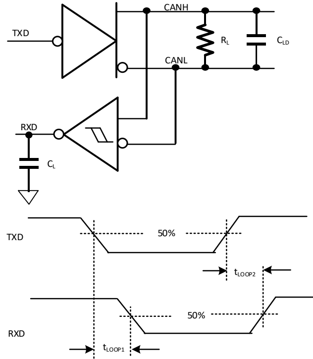
图 10-3 TXD 到 RXD 的环路延迟示意图
