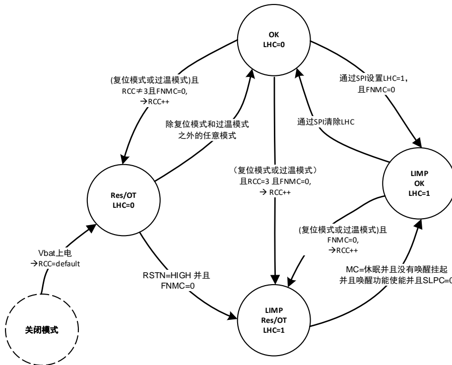
图 11-5 LIMP 状态机图
