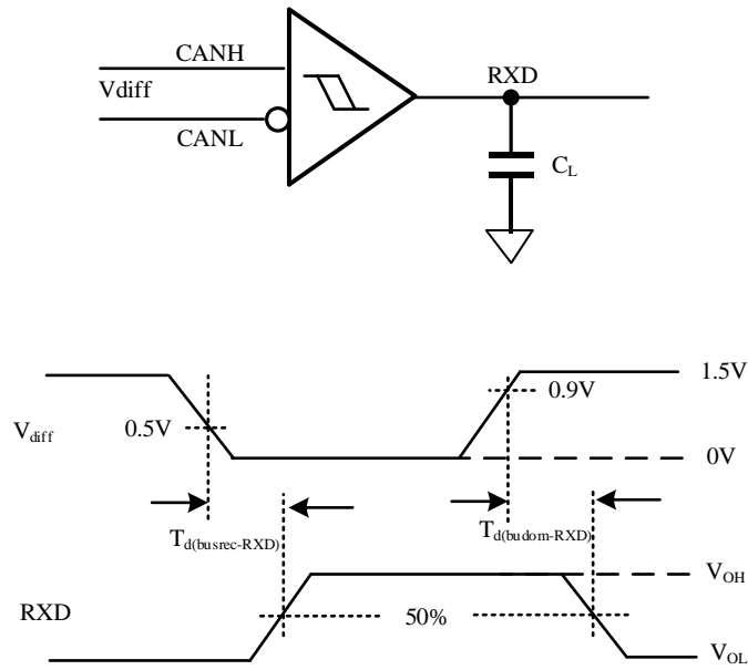
图 10-2 RXD 延迟示意图
