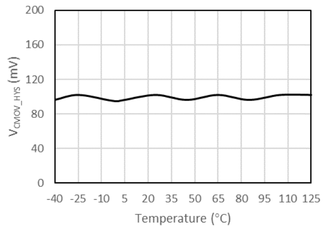
图 7-6 高边共模过压阈值迟滞窗口 vs 温度
