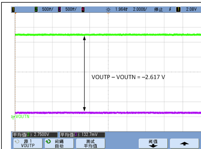
图 9-4 典型安全故障输出
