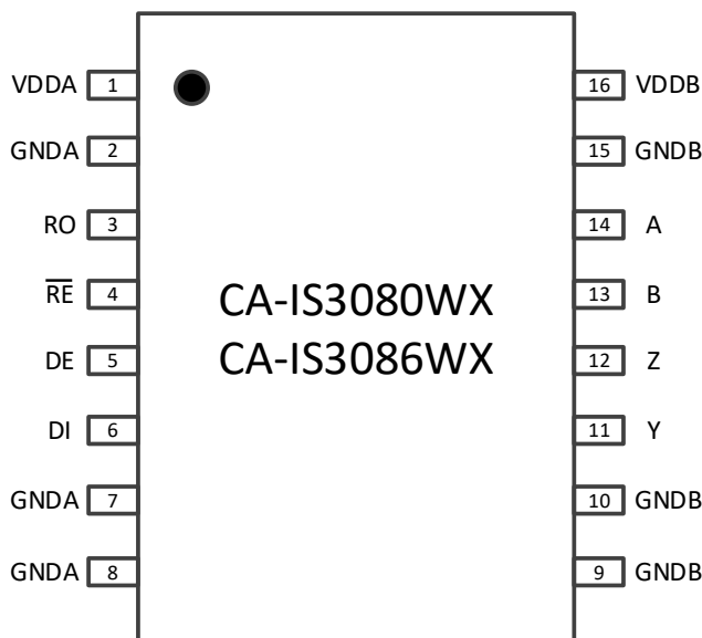
图 5-1 CA-IS3080WX 和 CA-IS3086WX 顶部视图
