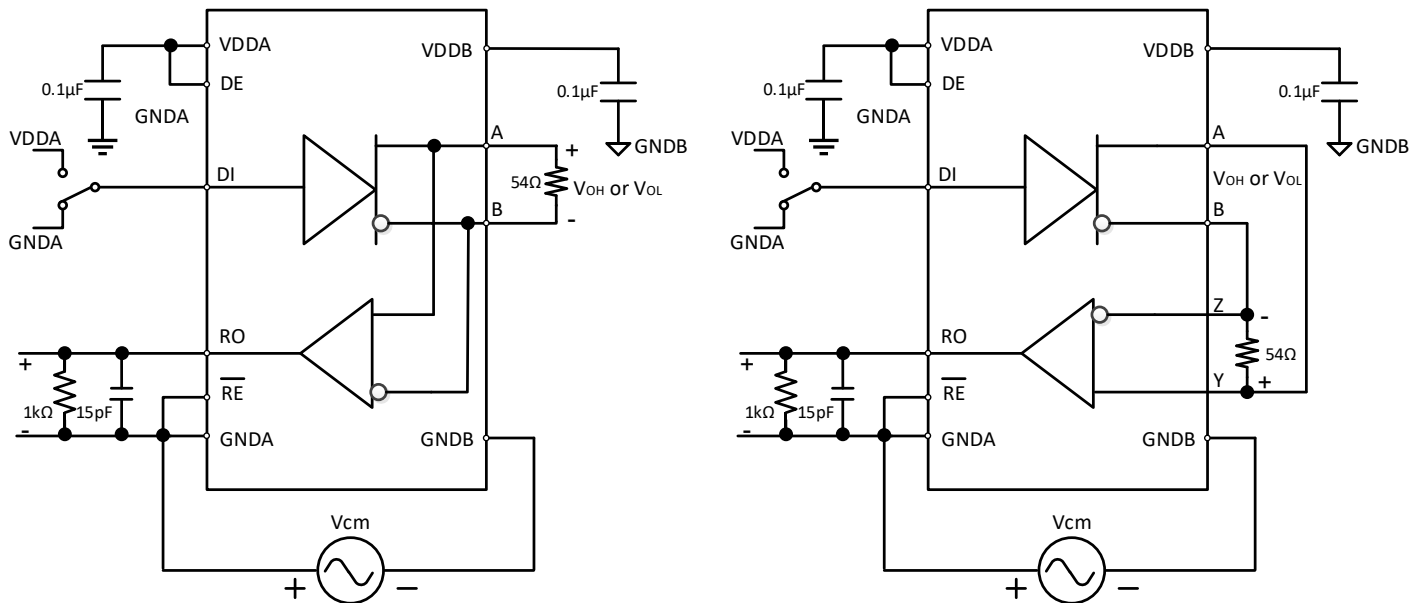
图 7-8 半双工（左）和全双工（右）收发器的共模瞬态抑制（CMTI）测试电路
