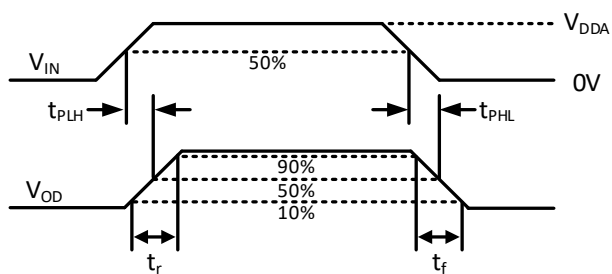
图 7-3 驱动器传输延时和上升下降时间
