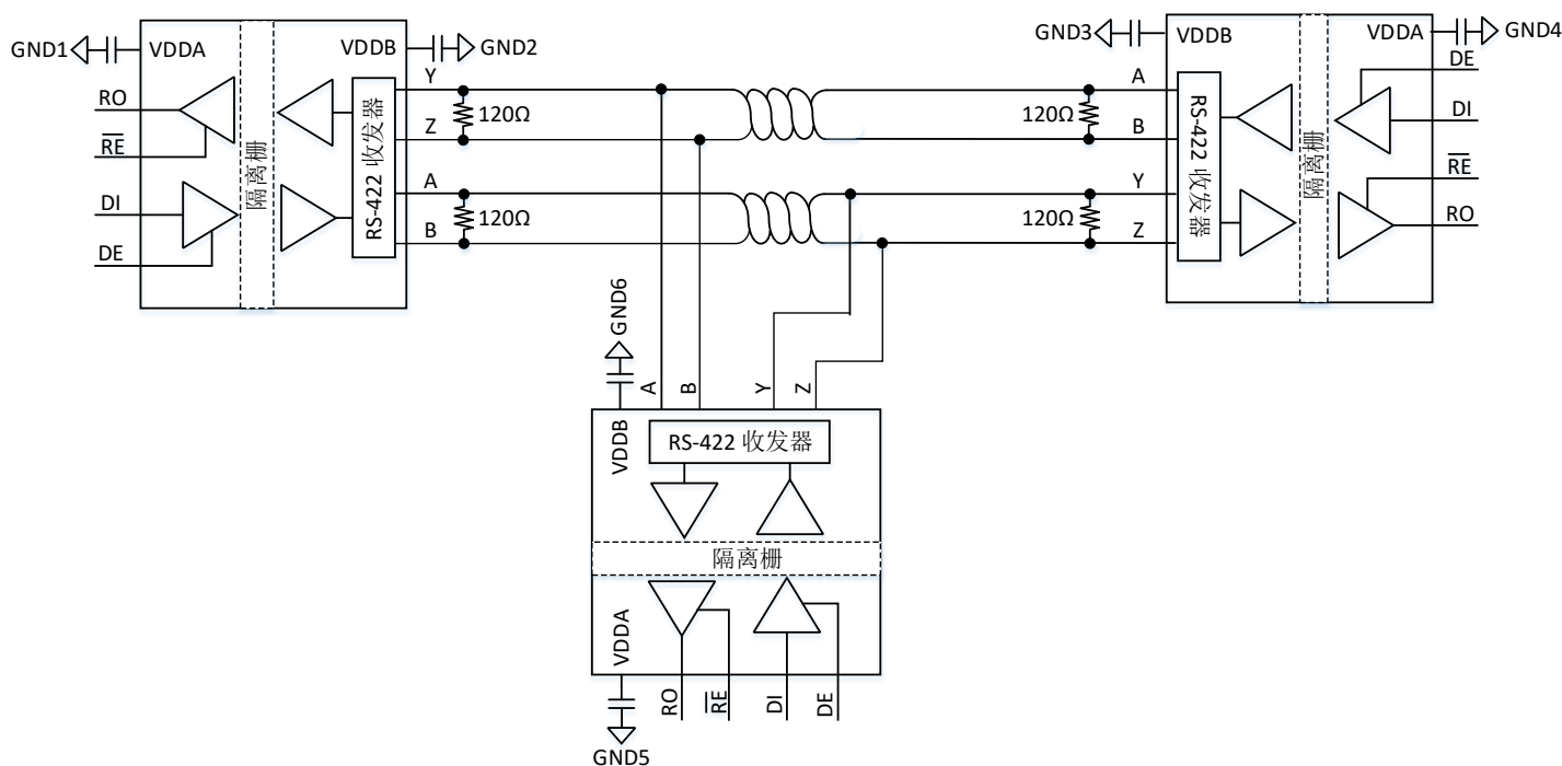
图 9-1 全双工 RS-422 网络架构示例
