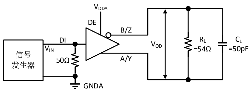
图 7-1 驱动器电压测试电路
