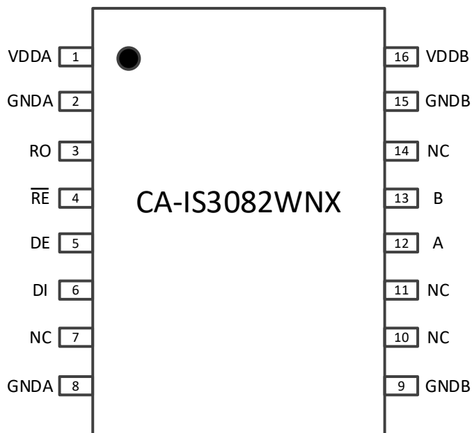
图 5-3 CA-IS3082WNX 顶部视图
