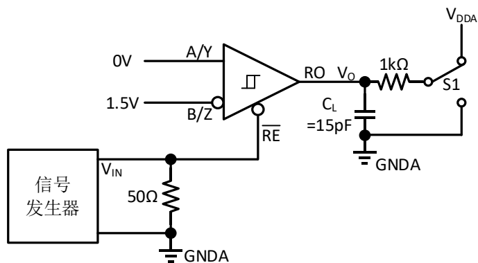
图 7-6 接收器开启和关闭时间
