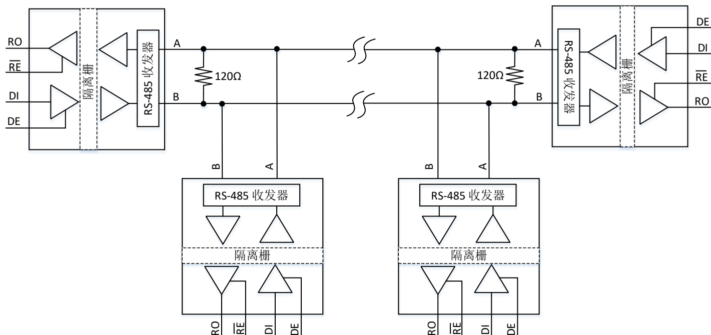
图 9-2 半双工 RS-485 网络架构示例
