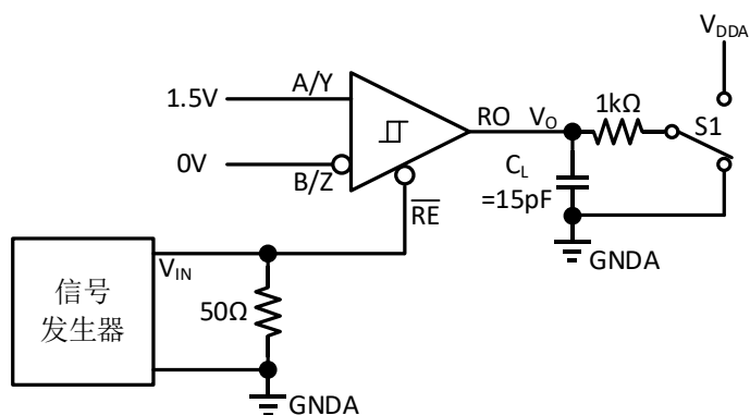
图 7-5 接收器传输延时和上升下降时间
