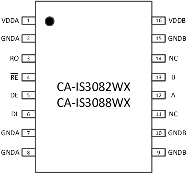
图 5-2 CA-IS3082WX 和 CA-IS3088WX 顶部视图
