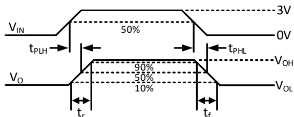
图 7-5 接收器传输延时和上升下降时间
