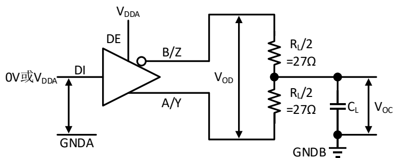
图 7-1 驱动器电压测试电路
