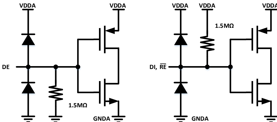
图 8-1 逻辑输入等效电路
