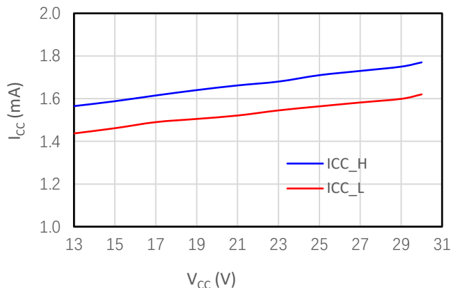
图 7-1 V_{CC} 供电电流 vs. V_{CC} 供电电压 @ 25^\circ C
