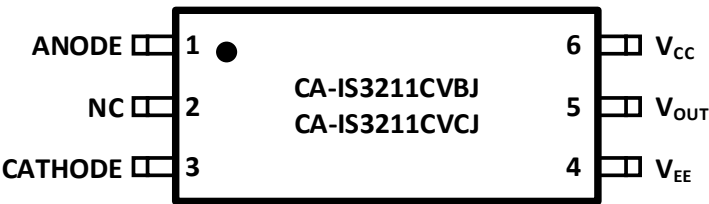
图 5-1 CA-IS3211CVBJ/CA-IS3211CVCJ 引脚配置
