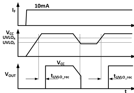
图 9-3 UVLO 功能
