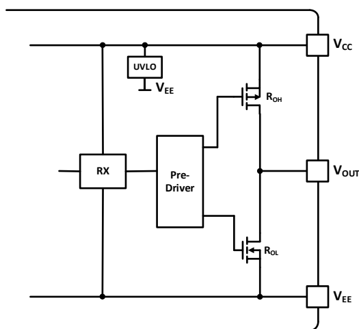
图 9-2 输出级结构
