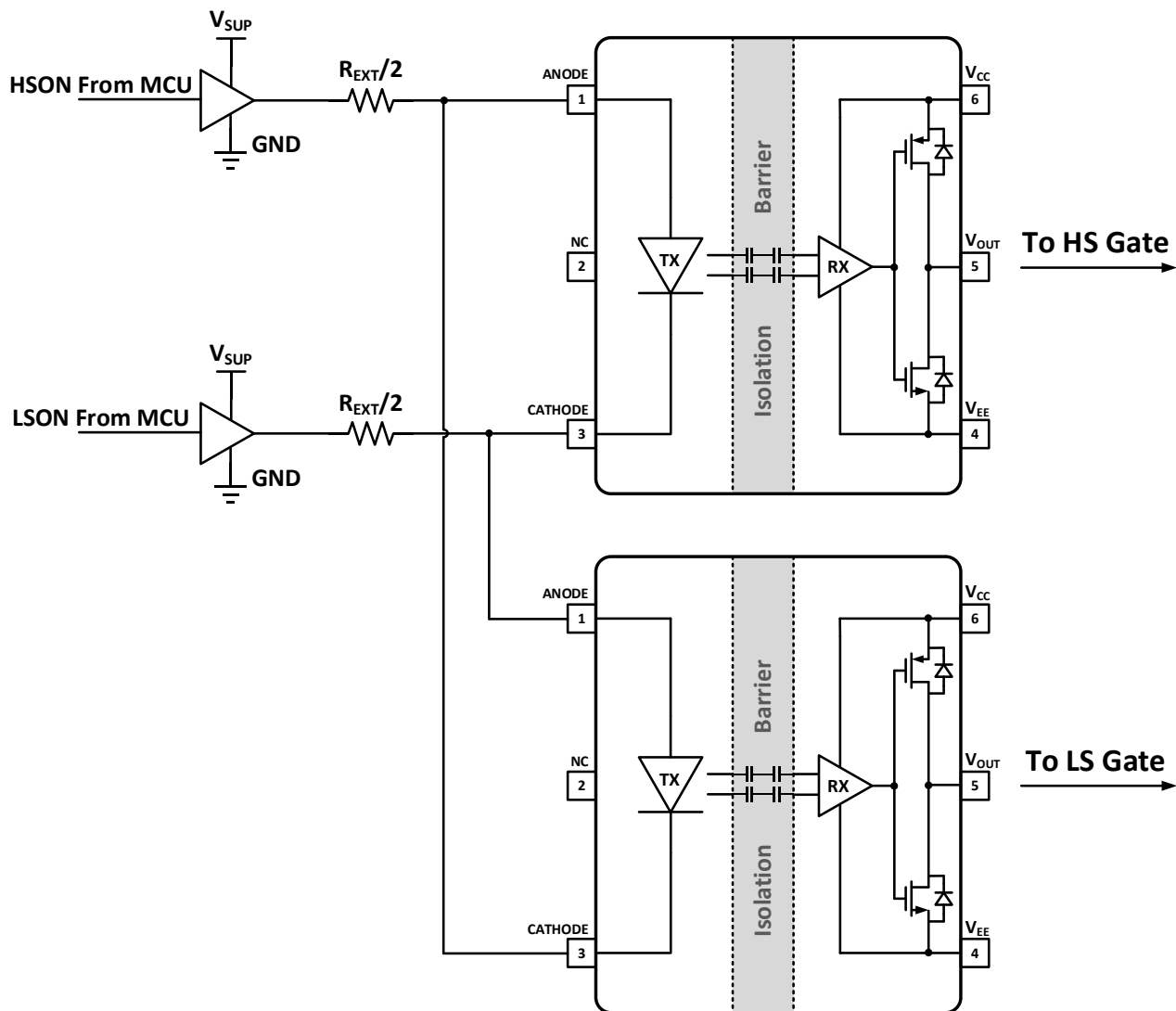
图 10-3 互锁配置
