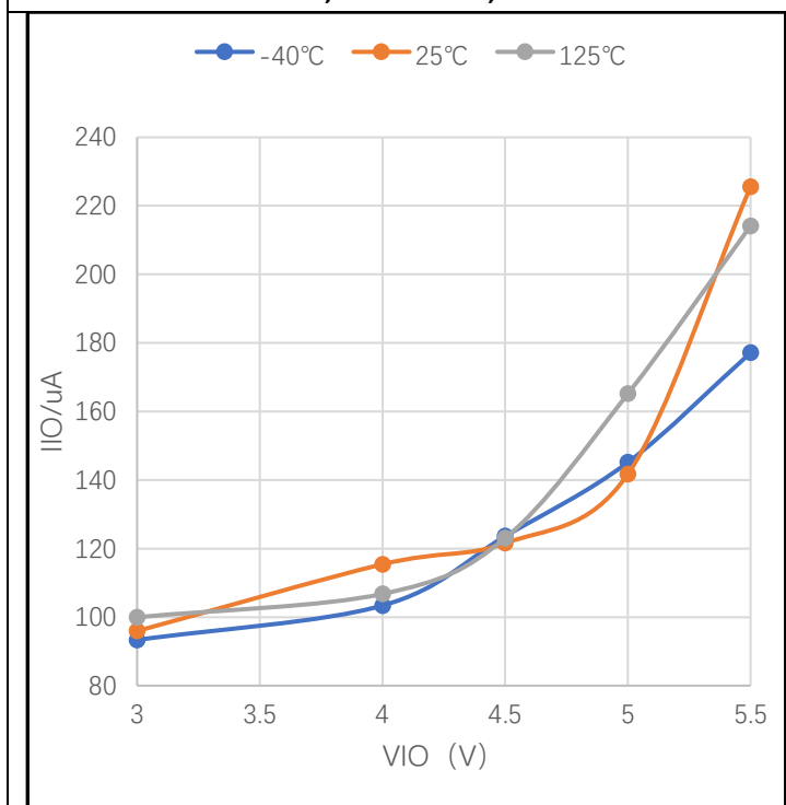
图 8-5 正常模式下 I IO 电流 (V CC =5V,TXD=STB=0V)
