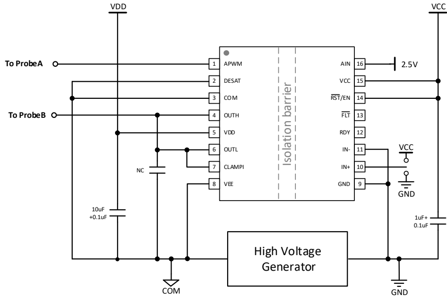
图 7-15 CMTI 测试方案 (CA-IS3217/8ANW-Q1)
