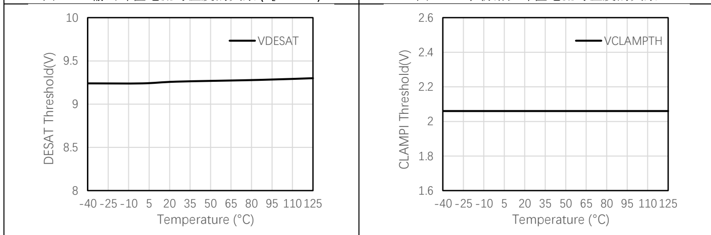
图 6-15 DESAT 阈值电压与温度的关系
