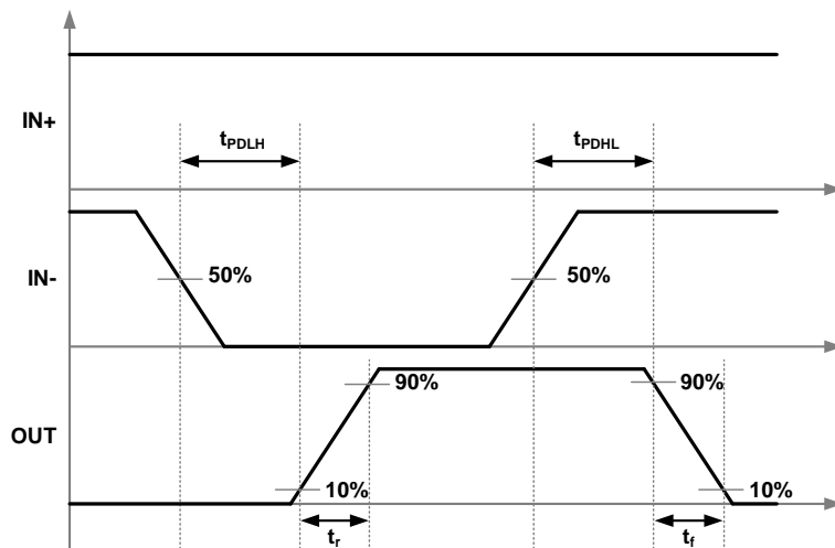
图 7-2 反相逻辑传播延迟测量
