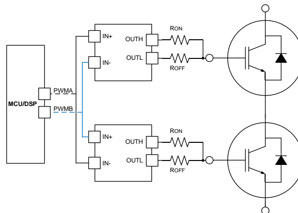
图 8-9 直通保护功能实际应用示意
