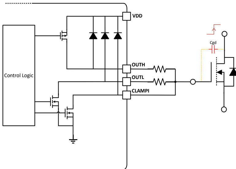
图 8-5 短路钳位
