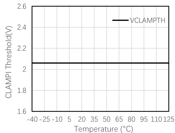
图 6-16 CLAMPI 阈值电压与温度的关系
