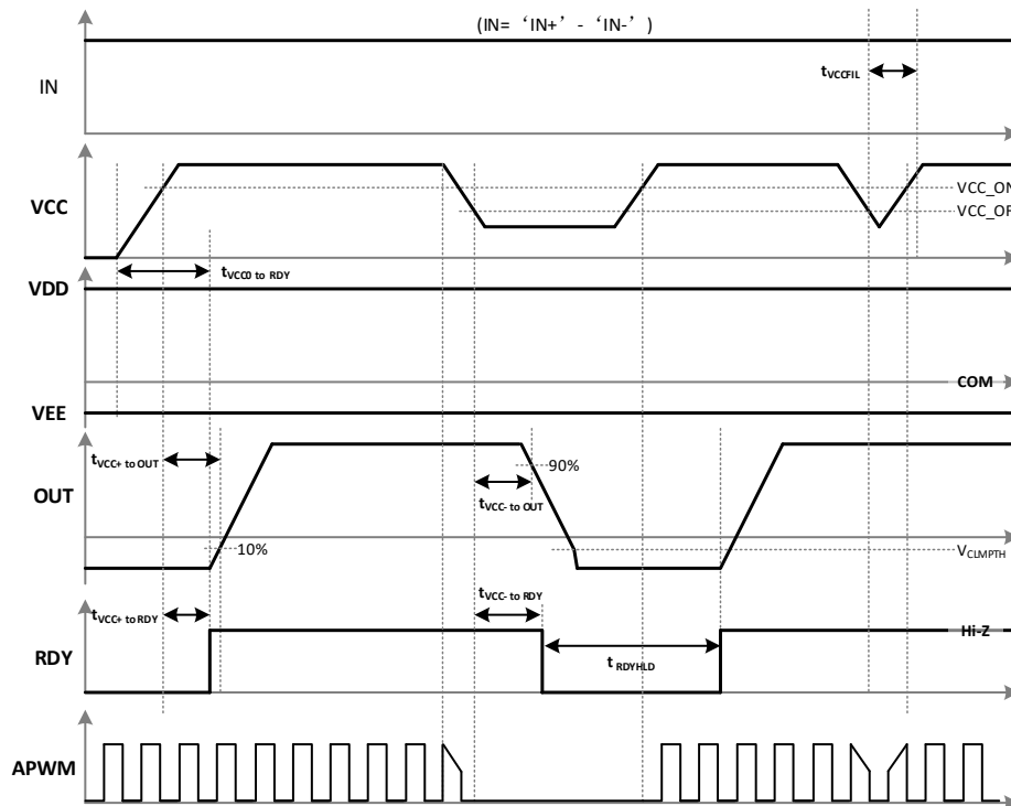
图 7-6 VCC UVLO 保护时序图
