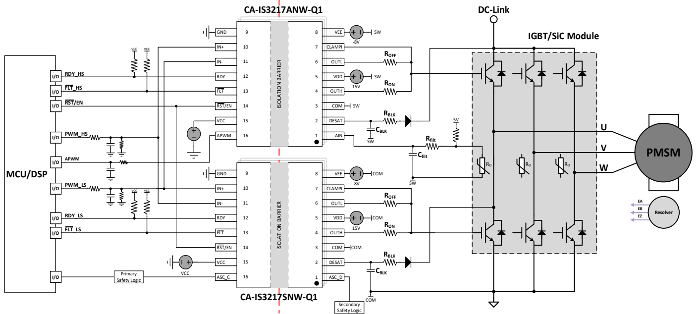
图 9-1 基于 CA-IS3217/8 驱动 IGBT/SiC 模块的典型三相电机应用
