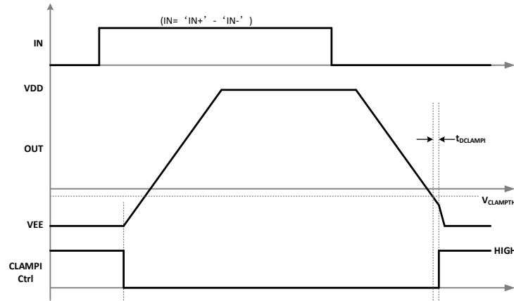
图 7-5 内置有源米勒钳位功能的时序图
