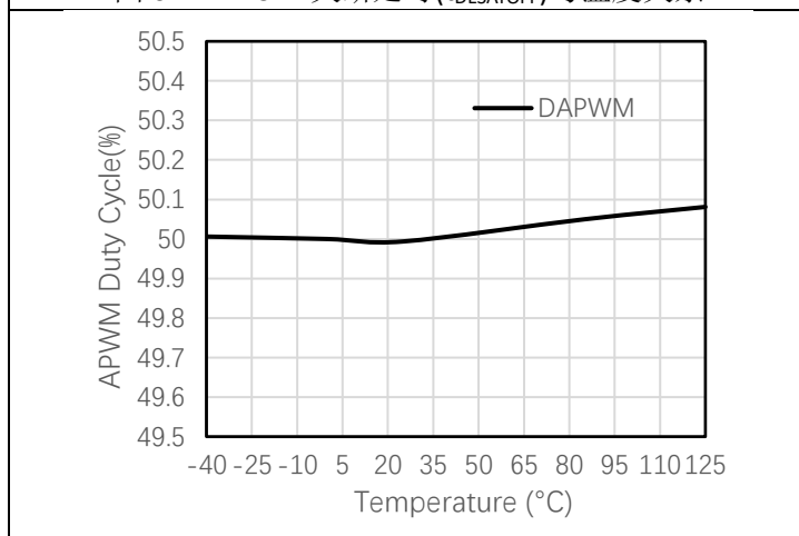
图 6-23 APWM 占空比与温度关系(AIN=2.5V)
