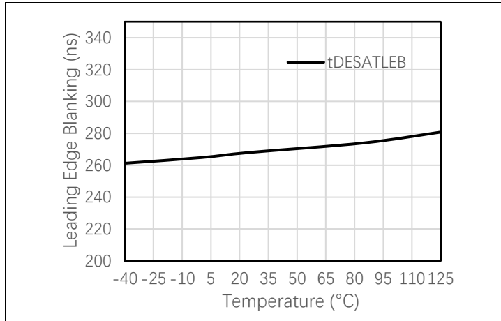
图 6-19 DESAT 消隐时间(t DESATLEB )与温度关系
