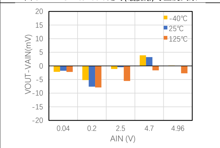
图 6-24 APWM 转换精度与 AIN 关系
