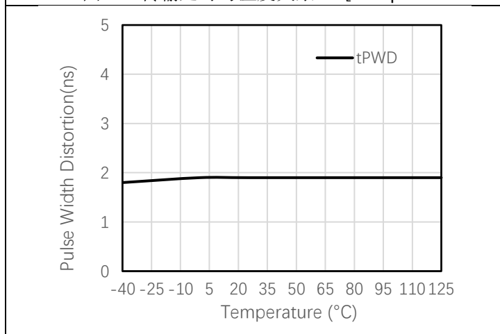
图 6-11 脉宽失真与温度关系
