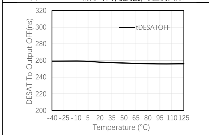
图 6-21 DESAT 关断延时(t DESATOFF )与温度关系
