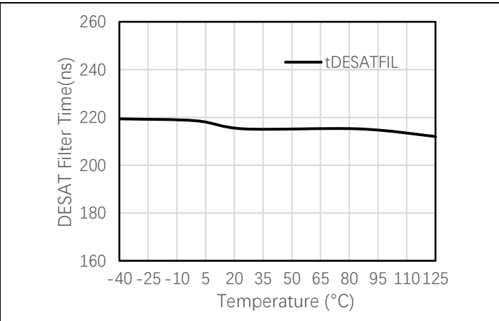
图 6-20 DESAT 滤波时间(t DESATFIL )与温度关系
