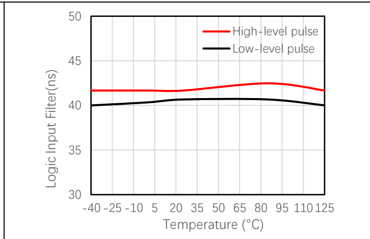
图 6-8 逻辑输入抗尖峰脉冲过滤时间与温度的关系
