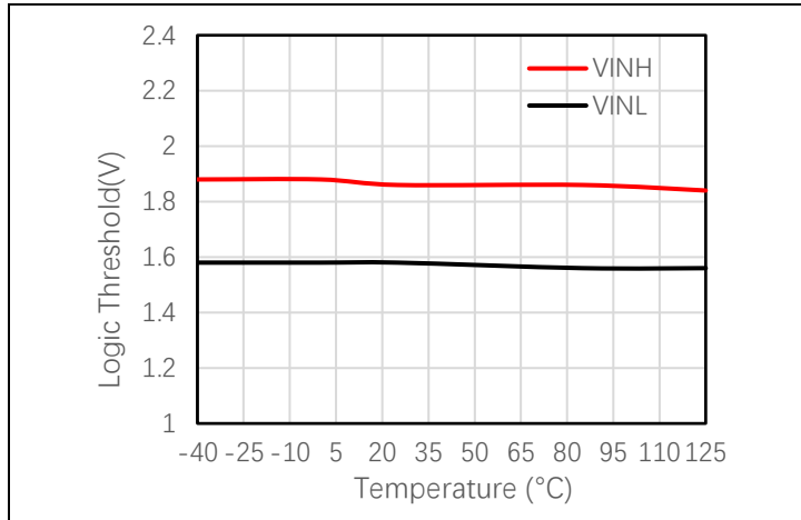
图 6-7 逻辑输入阈值与温度的关系
