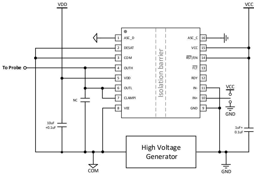
图 7-16 CMTI 测试方案 (CA-IS3217/8SNW-Q1)
