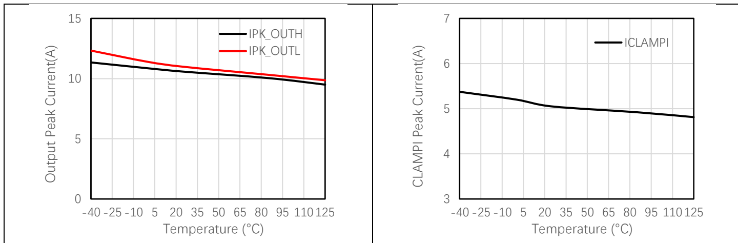
图 6-13 输出峰值电流与温度的关系 (C L =180nF)
