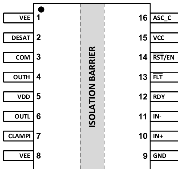
图 5-3 CA-IS3217/8LNW-Q1 引脚配置
