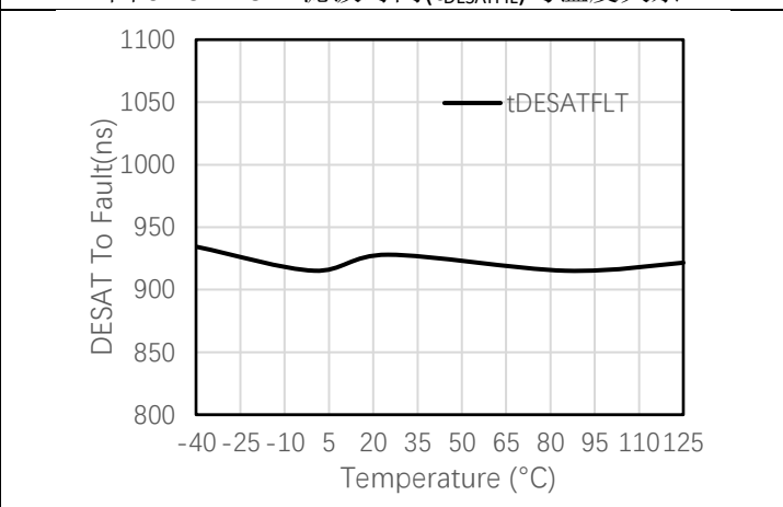
图 6-22 DESAT to Fault 延时(t DESATFLT )与温度关系
