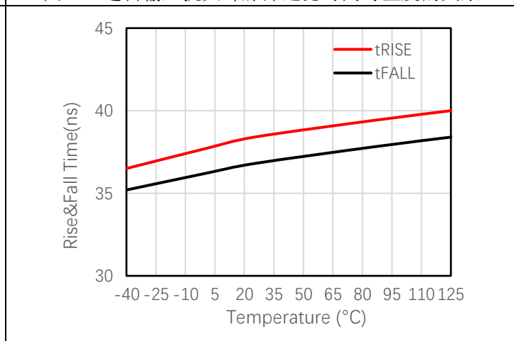
图 6-10 上升&下降时间与温度的关系 (C L =10nF)
