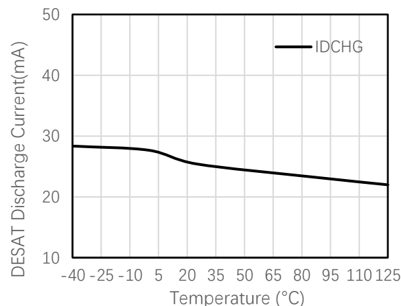
图 6-18 DESAT 放电电流(I DCHG )与温度关系
