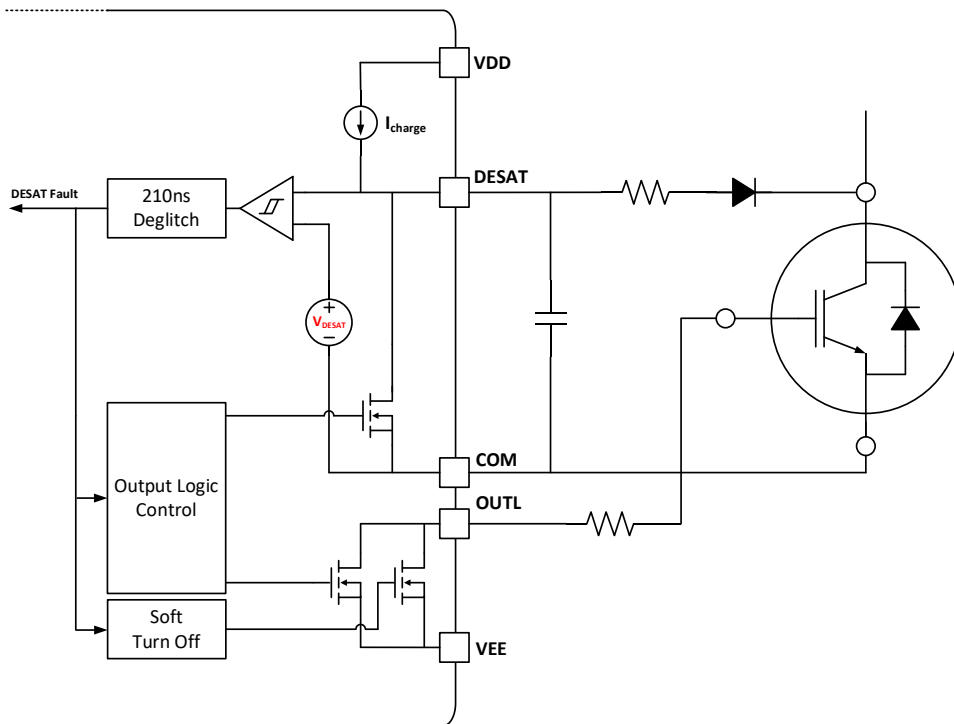
图 8-8 软关断
