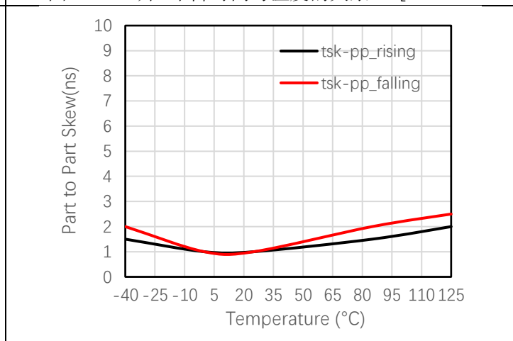
图 6-12 器件与器件之间的延时偏移与温度的关系
