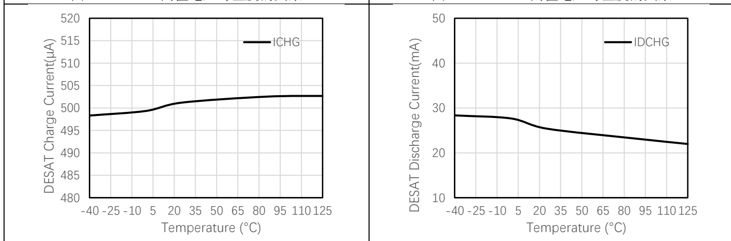
图 6-17 DESAT 充电电流(I CHG )与温度关系
