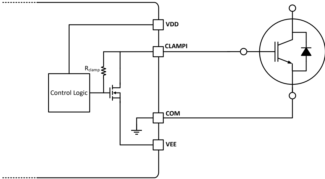
图 8-4 主动下拉
