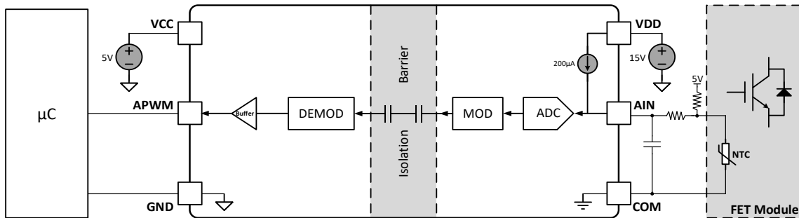
图 8-11 NTC 隔离采样电路图
