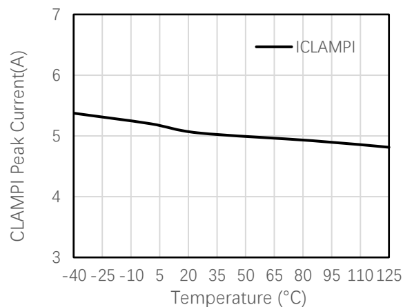
图 6-14 米勒钳位峰值电流与温度的关系
