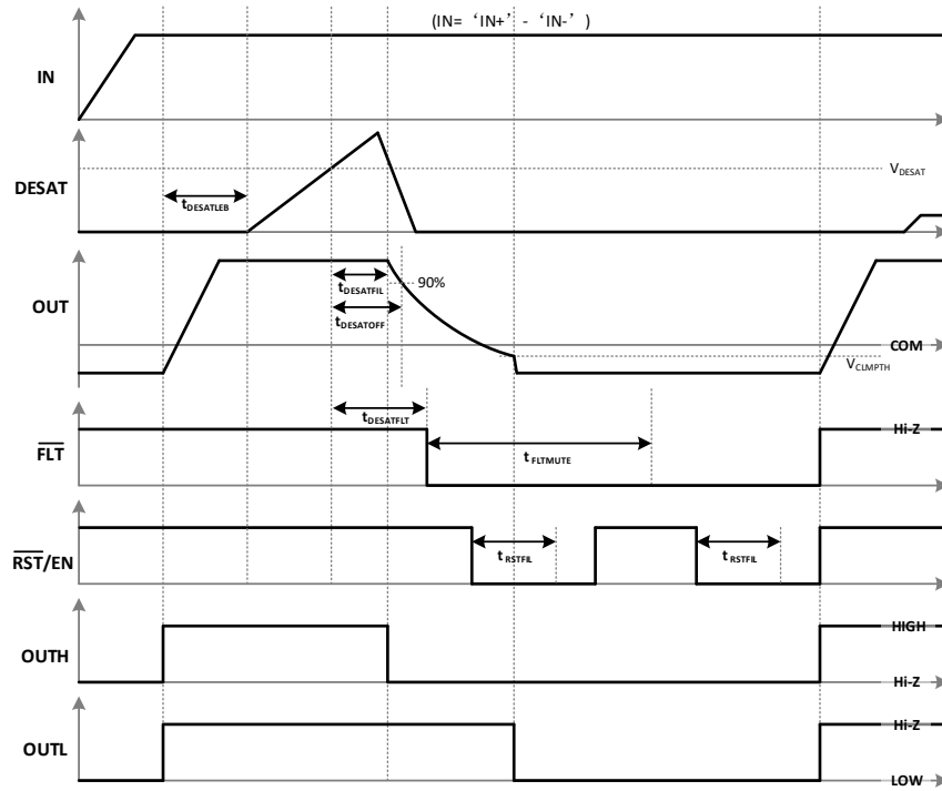
图 7-9 在开启转换期间带软关断功能的 DESAT 保护
