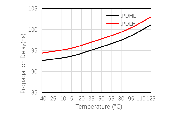
图 6-9 传输延时与温度关系 (C L =100pF)
