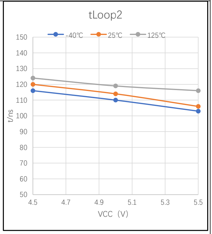
图 8-114 Loop2 Delay
