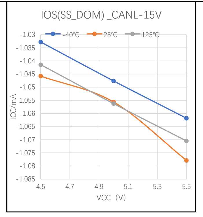
图 8-10 CANL 短路电流 (VIO=VCC,CANL=-15V)
