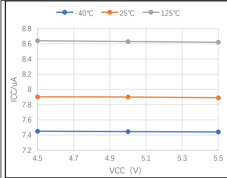
图 8-1 待机状态 I_{CC} 电流 (VIO=VCC, STB=VCC, RL=50 Ω)
