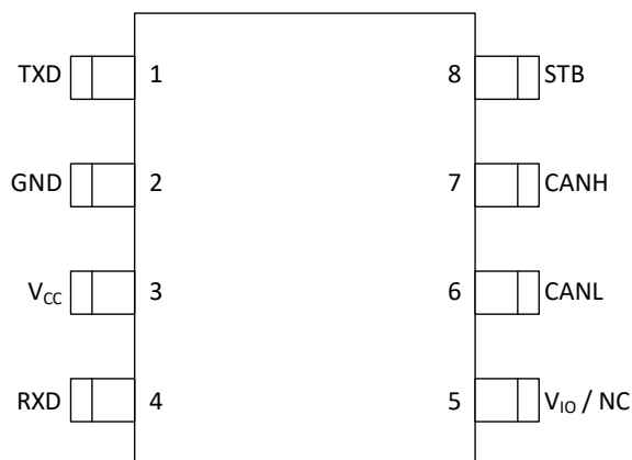
图 5-1 CA-IF1044Ax 引脚图
