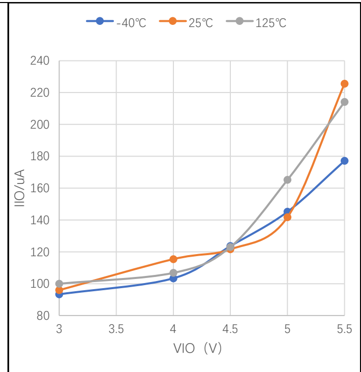
图 8-5 正常模式下 I IO 电流 (V CC =5V,TXD=STB=0V)
