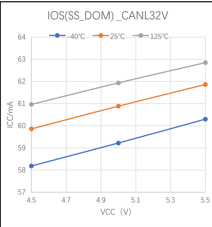
图 8-9 CANL 短路电流 (VIO=VCC,CANL=32V)
