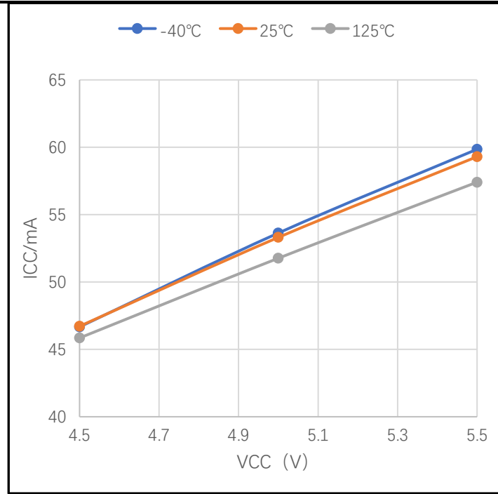
图 8-3 50Ω 负载下显性状态 I cc 电流 (V IO =V CC ,STB=V CC =0v,RL=50 Ω)
