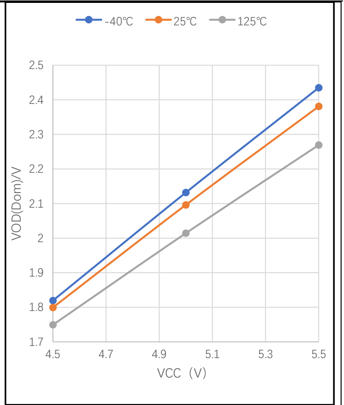
图 8-112 60Ω 负载下差分输出电压 (VCC=VIO)
