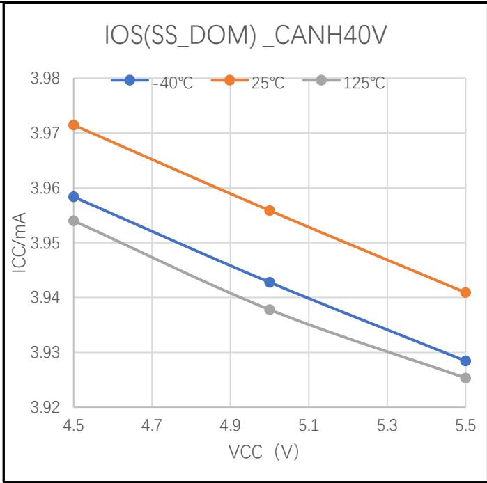
图 8-7 CANH 短路电流 (VIO=5V,CANH=40V)
