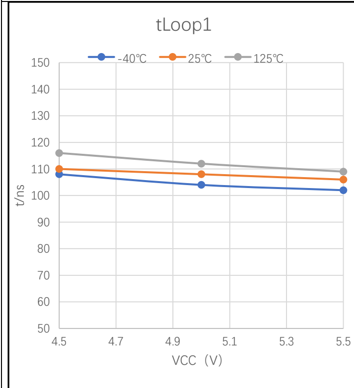
图 8-113 Loop1 Delay
