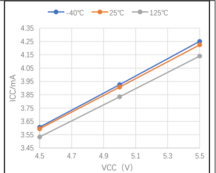
图 8-2 隐性状态 I_{CC} 电流 (VIO=VCC, STB=VCC, RL=50 Ω)
