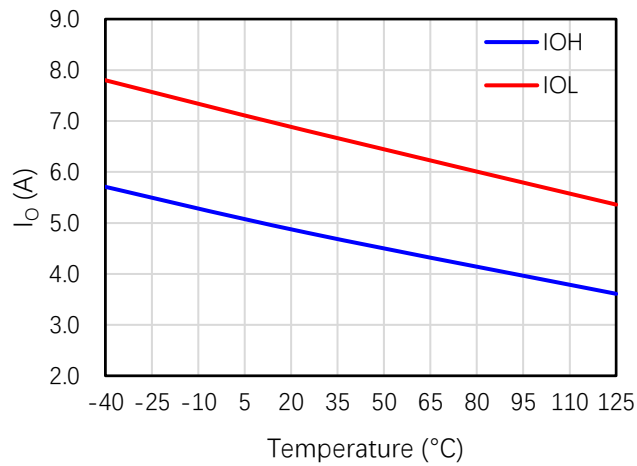
图 7-6 输出峰值电流 vs. 温度
