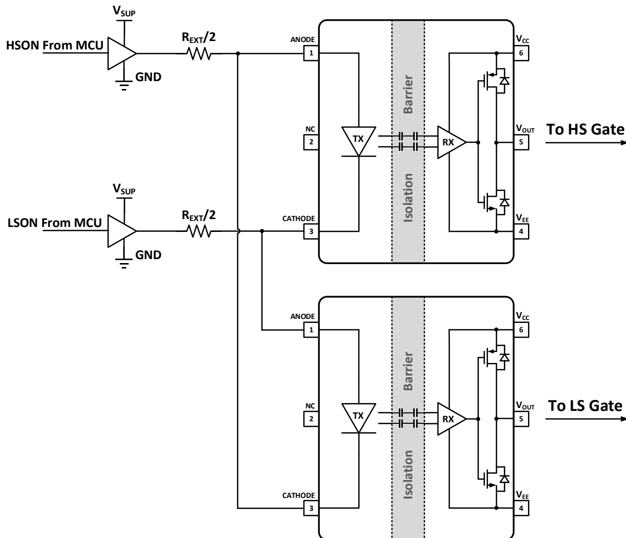
图 10-3 互锁配置
