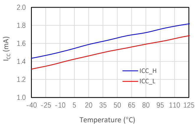
图 7-2 V_{CC} 供电电流 vs. 温度
