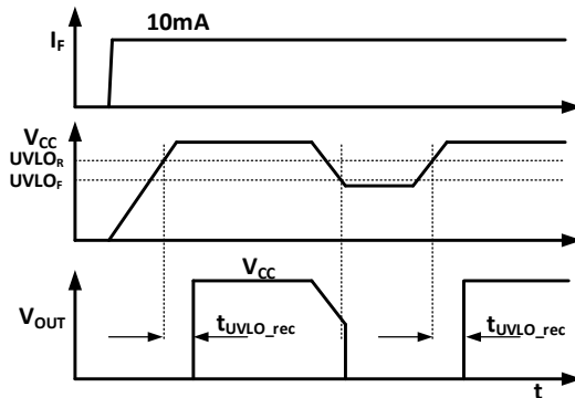
图 9-3 UVLO 功能
